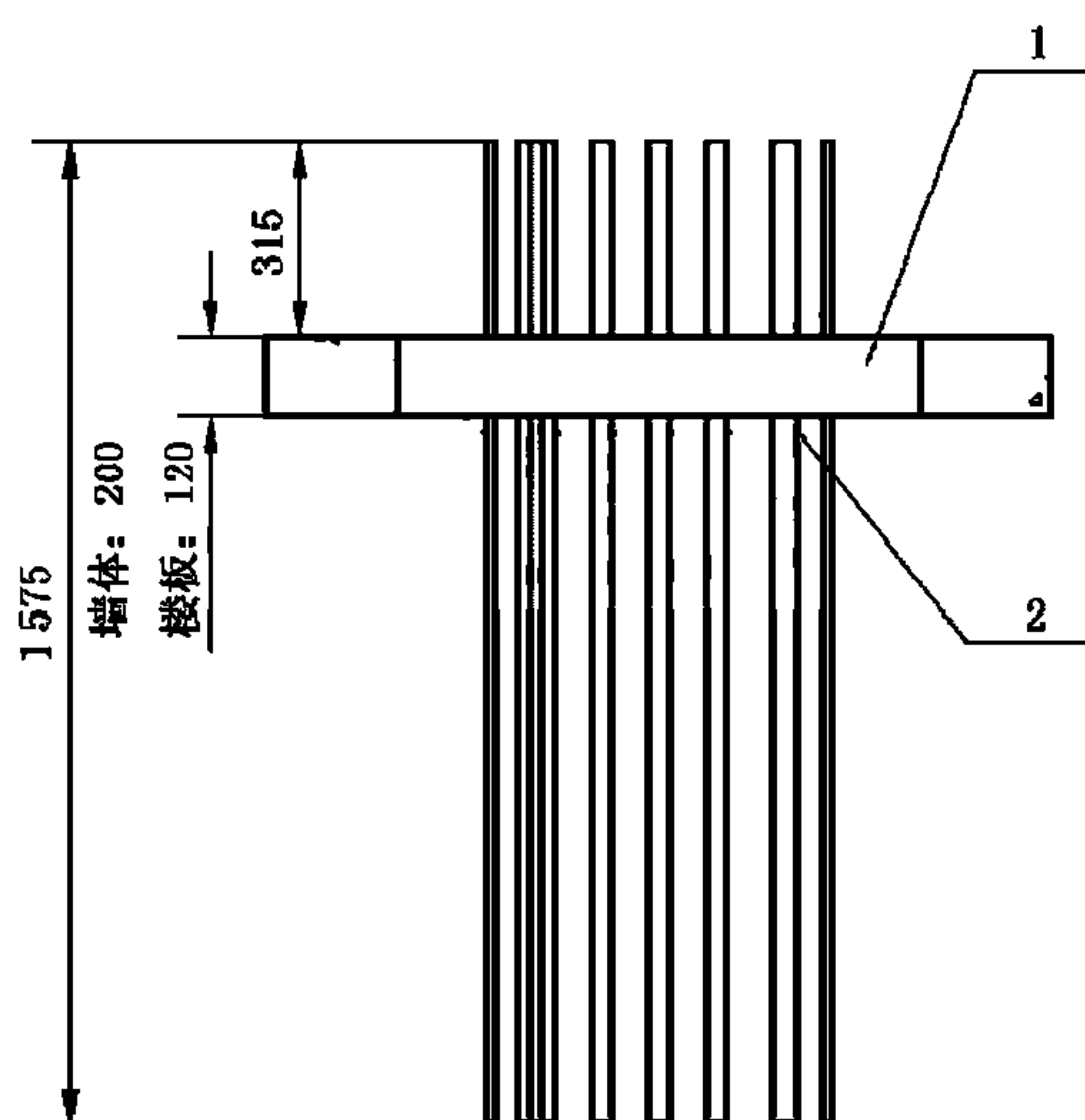
俯视图
